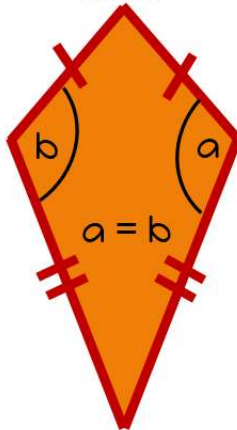
Vlieër
