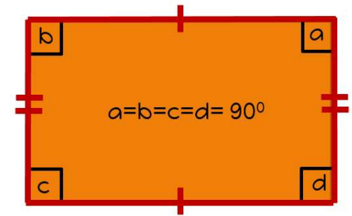
Reghoek
