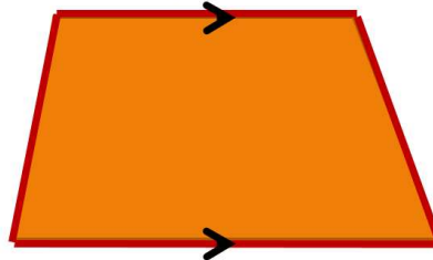
Trapesium
