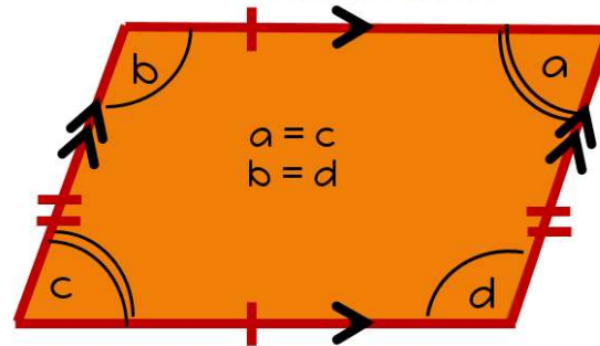
Paralellogram
