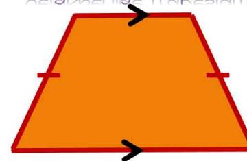
Gelykbenige Trapesium
