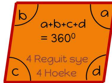
Vierhoek
